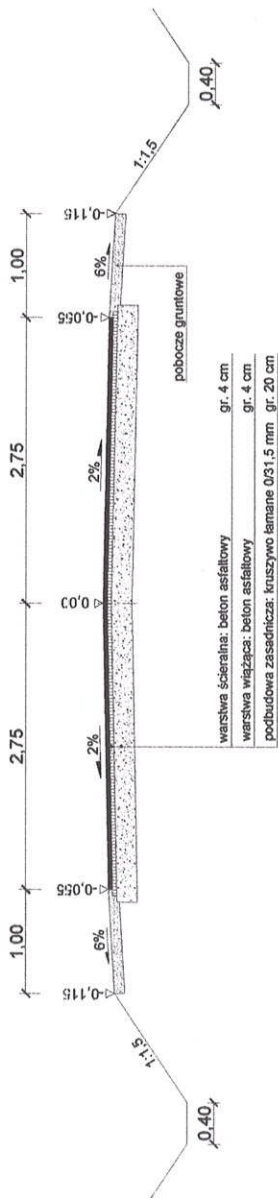
przekrój na odcinku od km 1+780 do km 2+590 za wyjątkiem łuku o R=155 m
